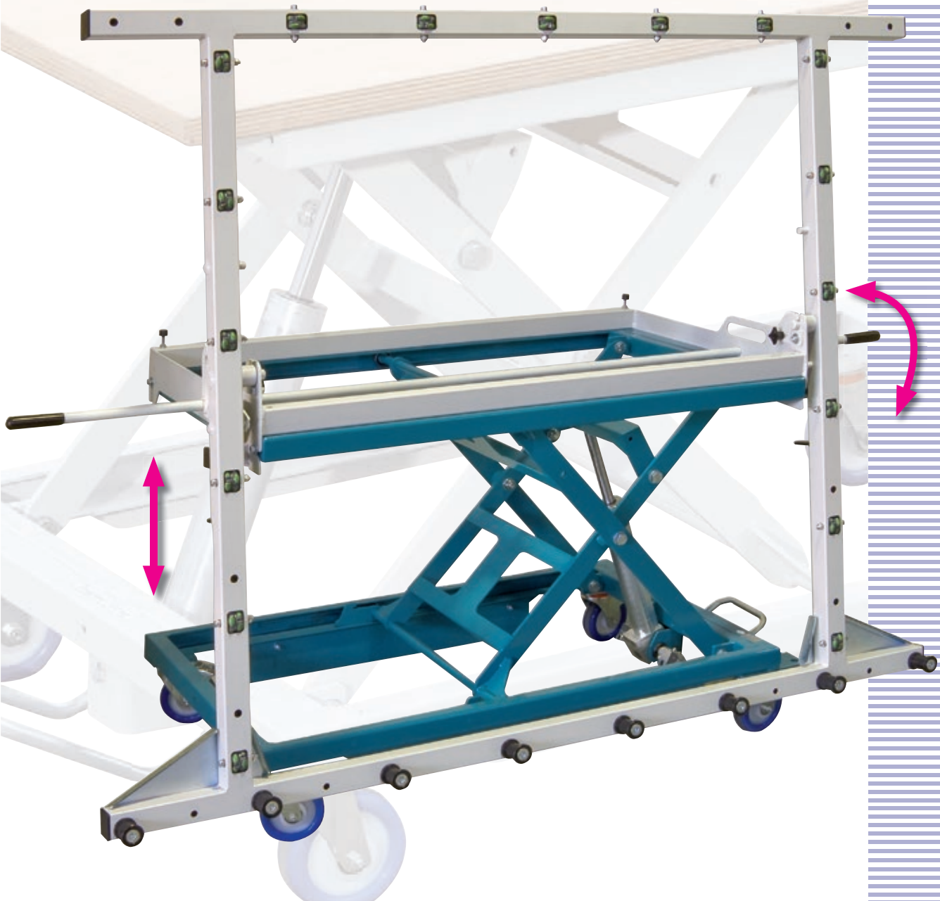
NIVEAU HS 300-midi mit Plattformschwenkrahmen
